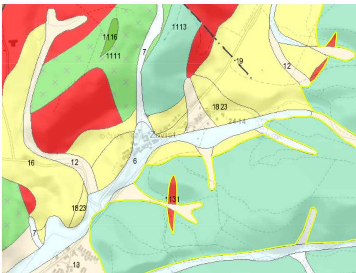
Obrázek 22: Geovědní mapa obce 24
