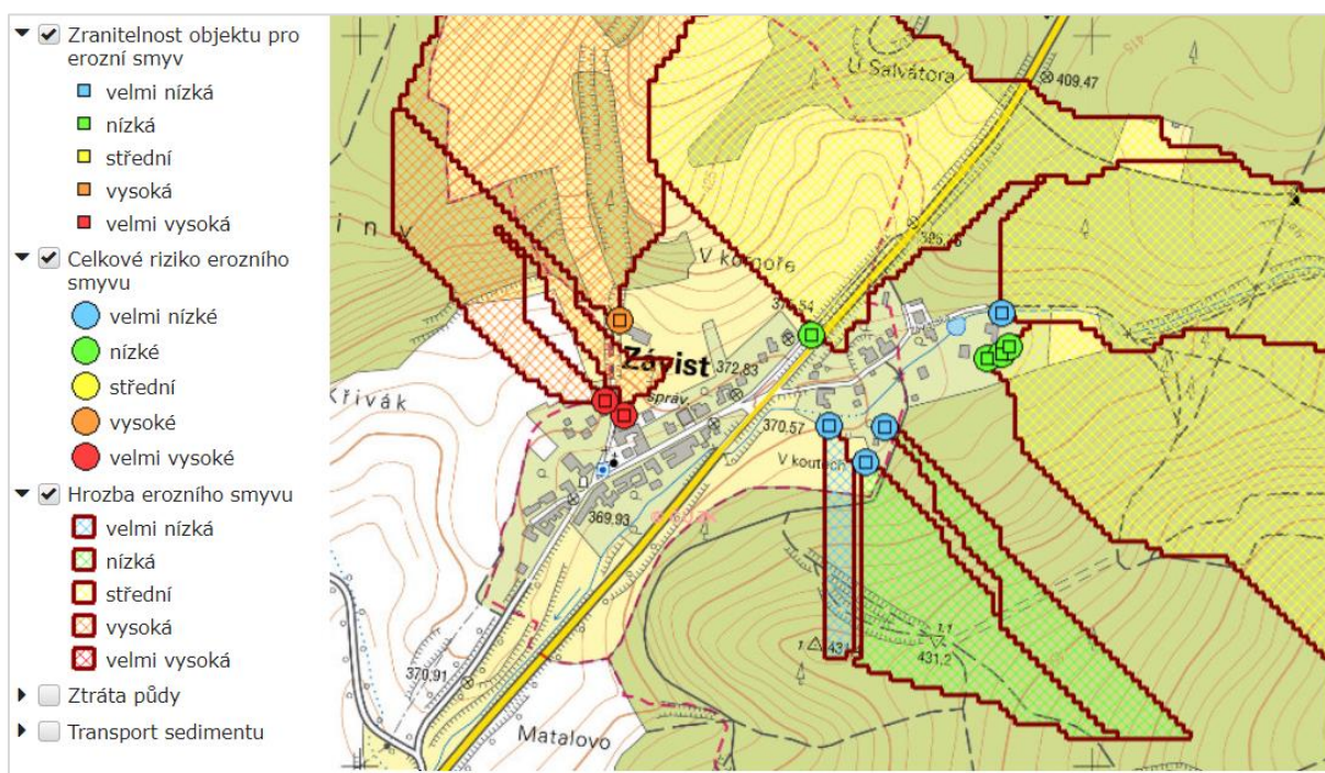
Obrázek 18: Hrozba erozního smyvu 25
